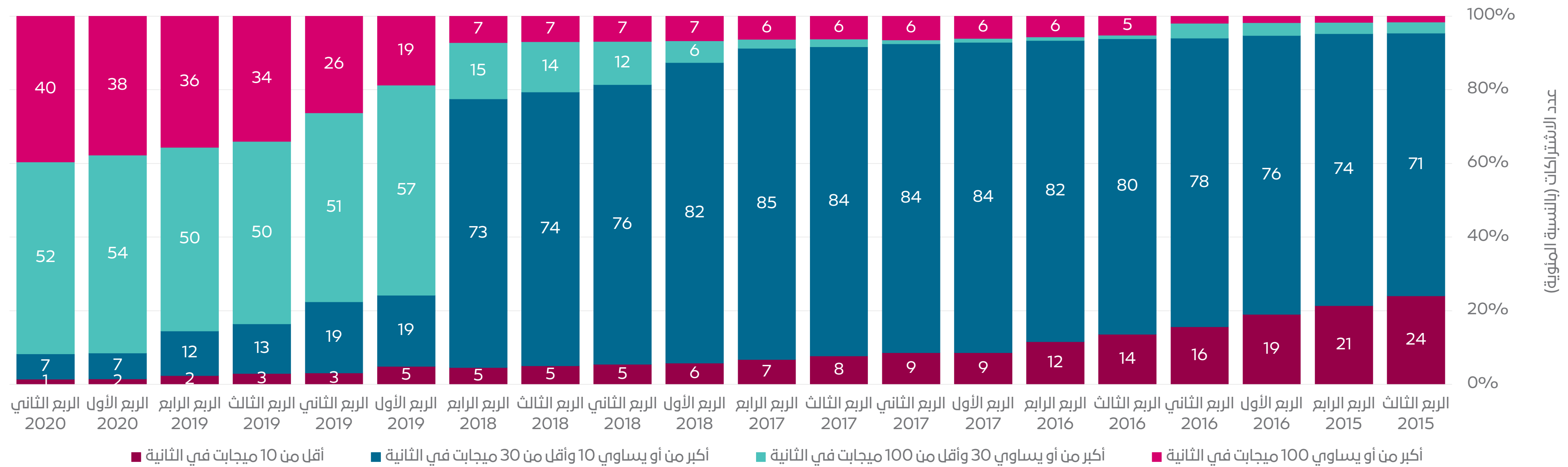
أعداد الاشتراكات في خدمات البرودباند الثابت حسب السرعة (بالنسبة المئوية)
